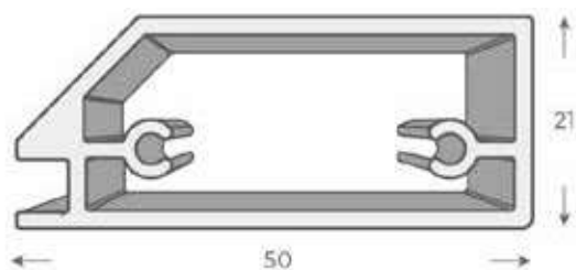
Perfil: Vertical
