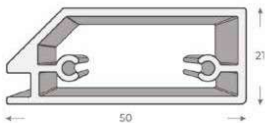
Perfil: Vertical
